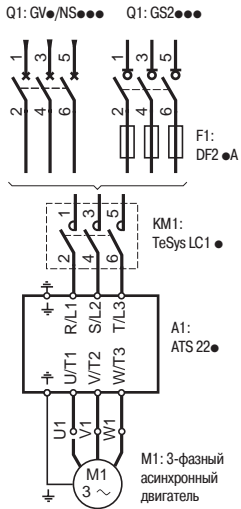
Altistart 22, защищаемый автоматическим выключателем или разьединителем
